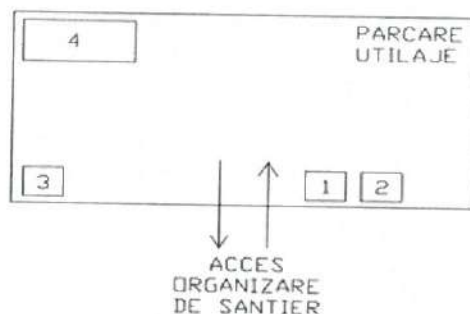
Fig. 17. Model de organizare de șantier
