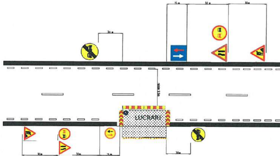
Fig. 11 –semnalizare lucrari parte carosabila si trotuar
